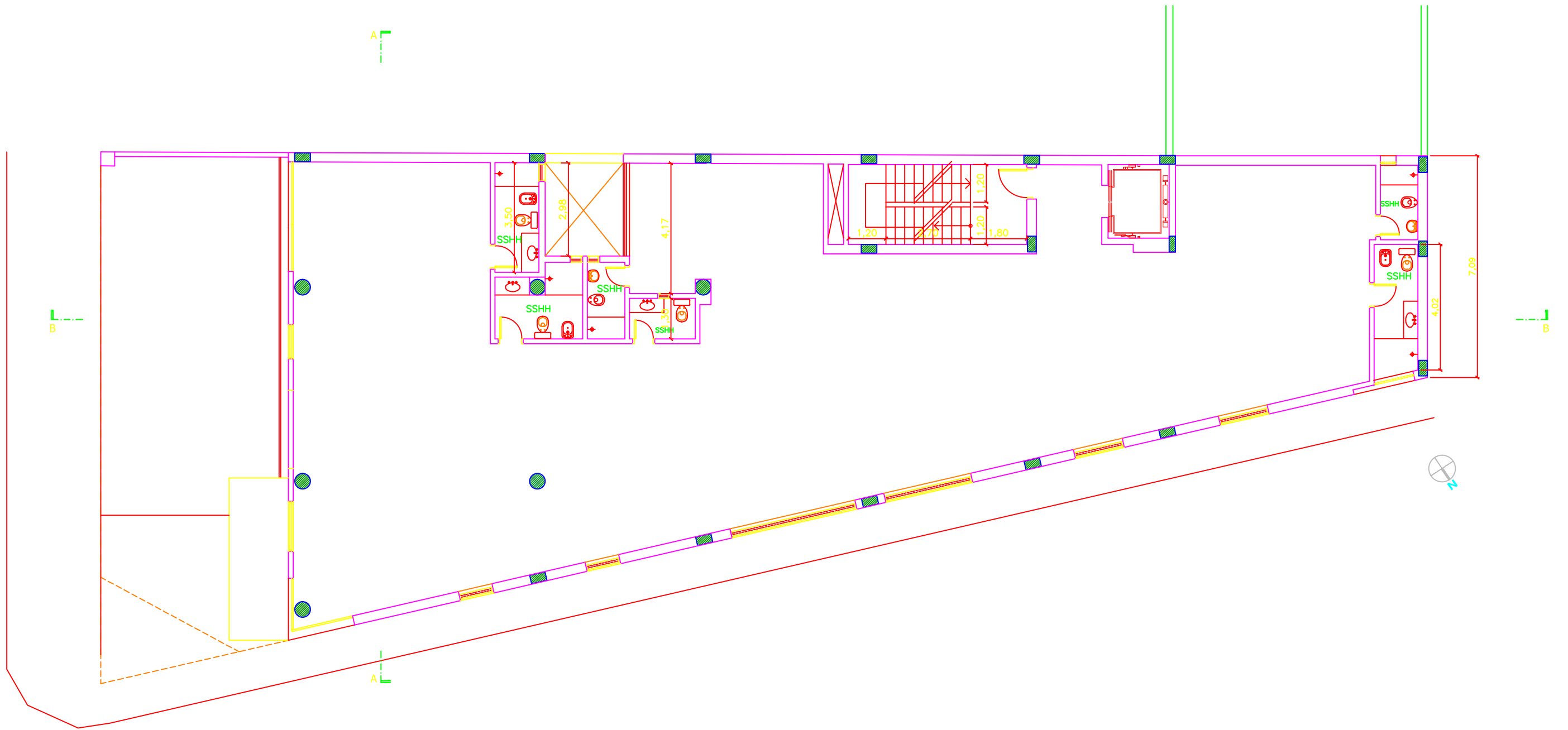
PLANTA ARQUITECTÓNICA – NIVEL +6,72 y 10,32 Escala 1:100
