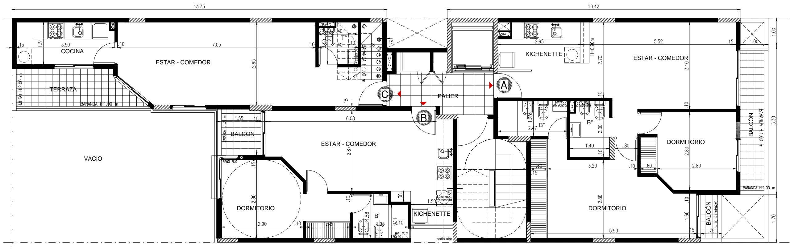
Planta 5° piso
