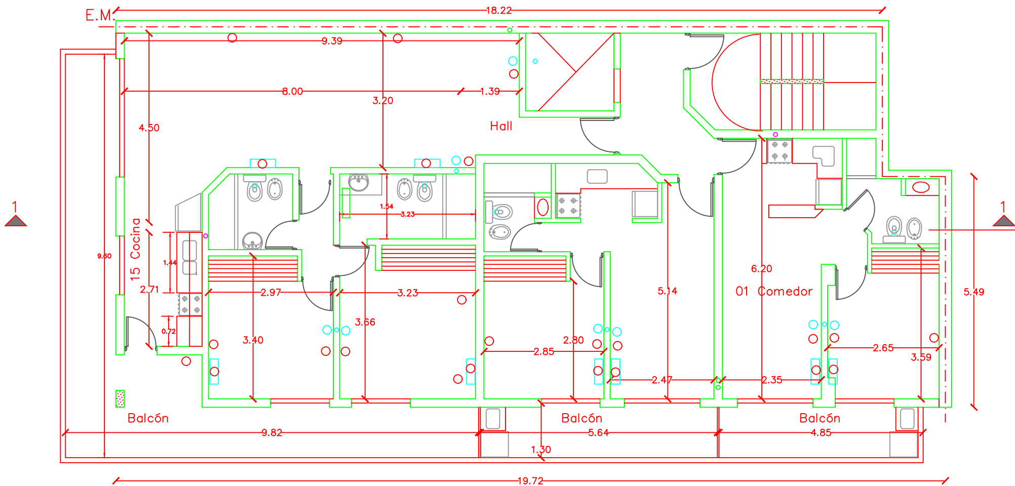
PLANTA TIPO OFICIAL Y DEFINITIVA DEL 2so AL 8vo
