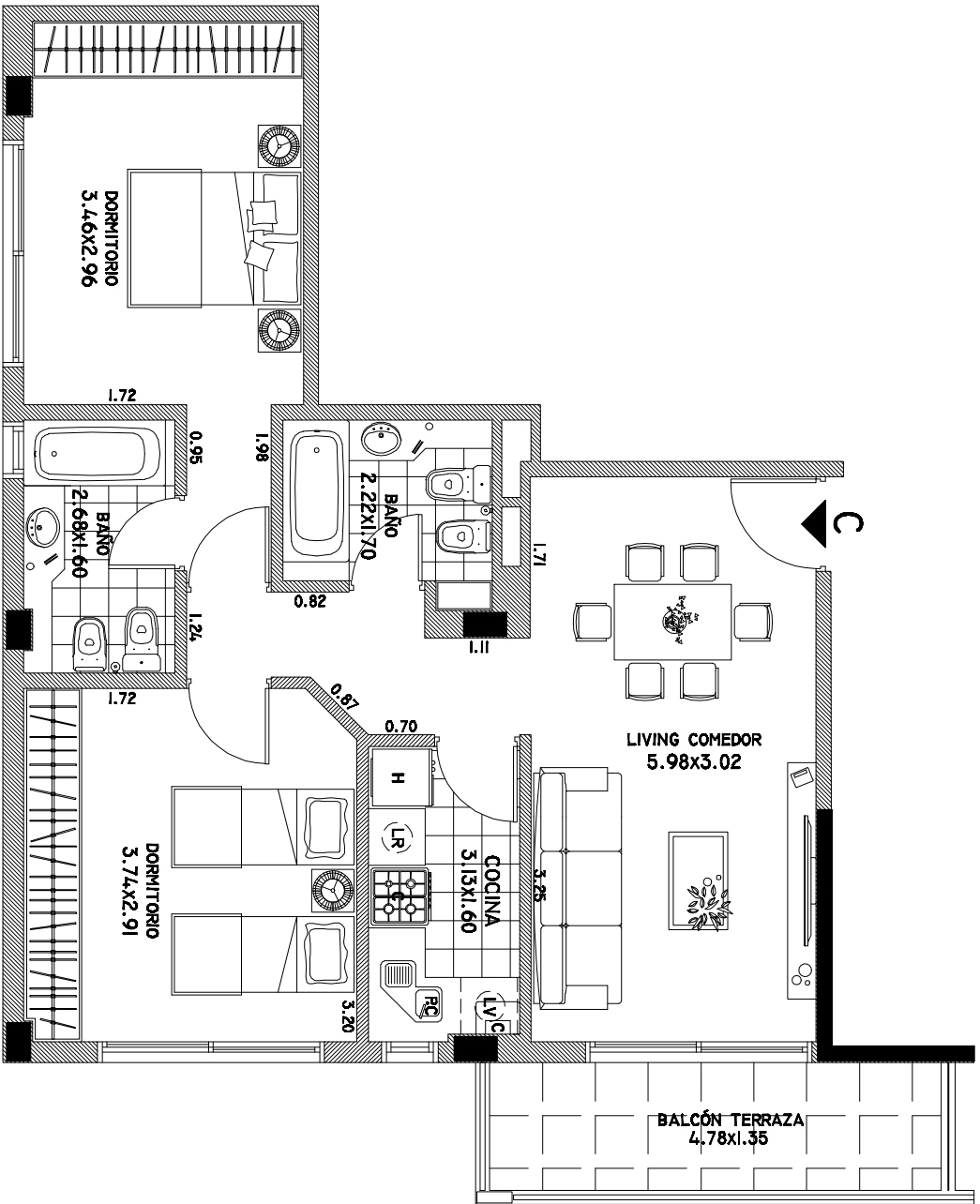
PLANTA PISO 1/3 - DEPTO (C) ESC 1:75
