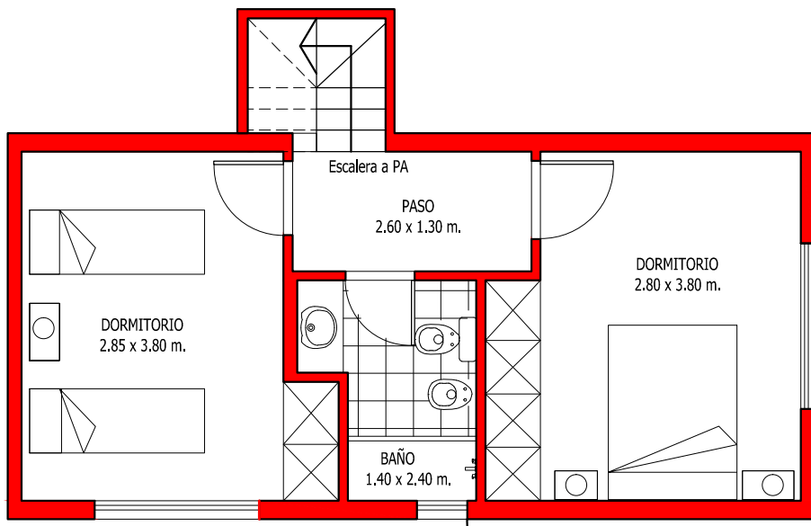
DEPTO 301 - ENTREPISO
