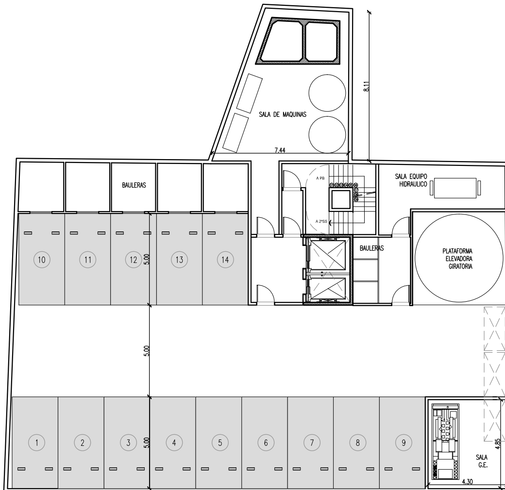
2º SUBSUELO ESC. 1:200
