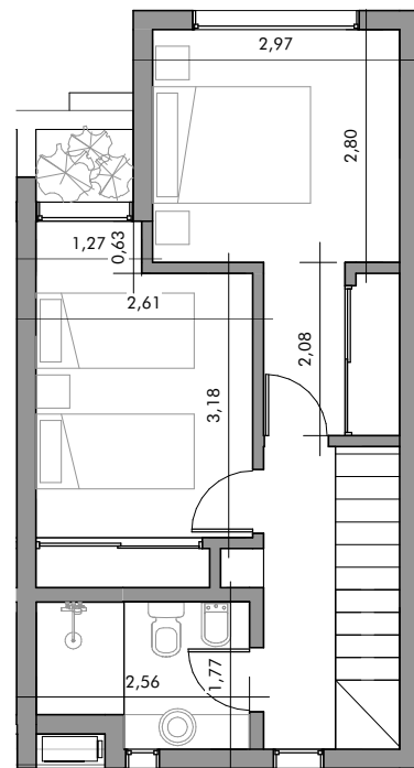
PLANTA ALTA
