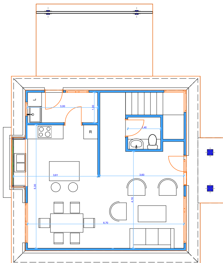
0. PLANTA BAJA 1:100
