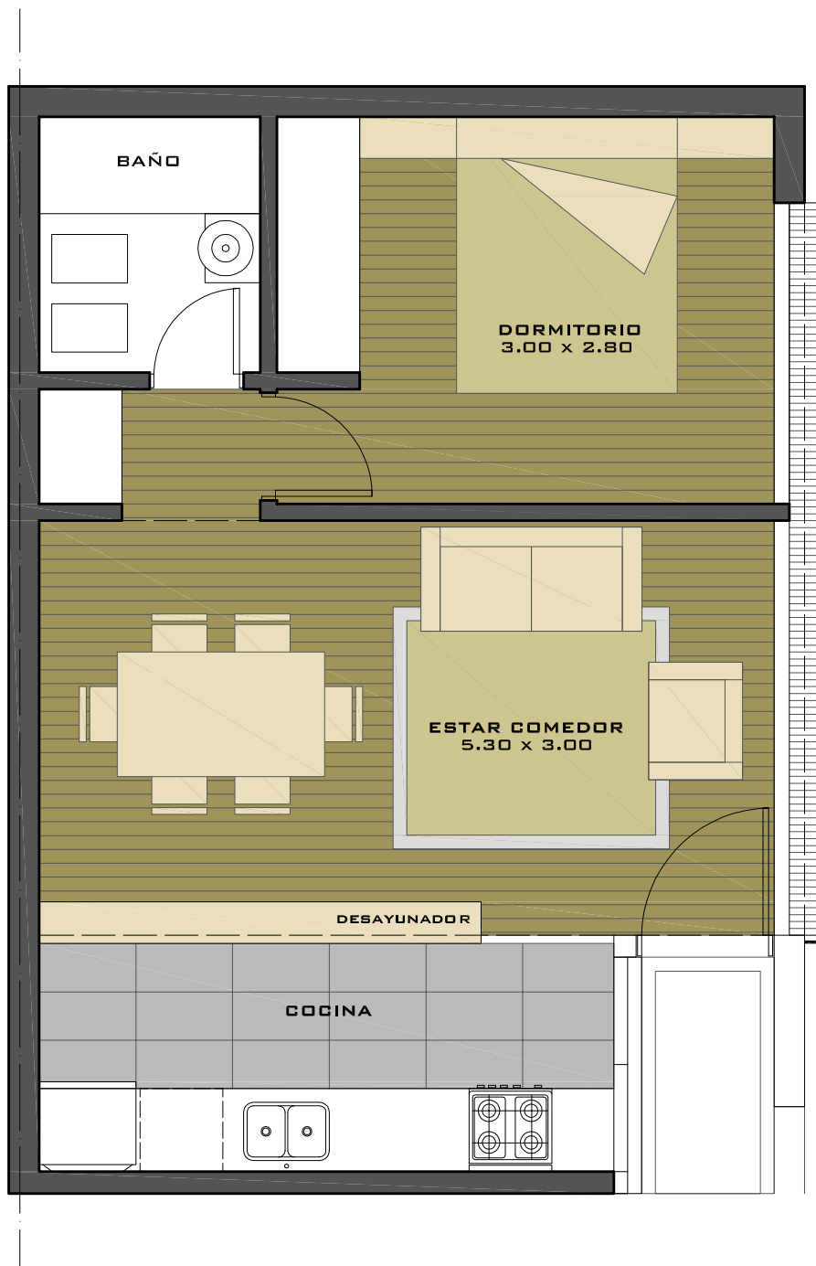
UNIDAD DE 2 AMBIENTES - DPTO. PB "005" y "013"
