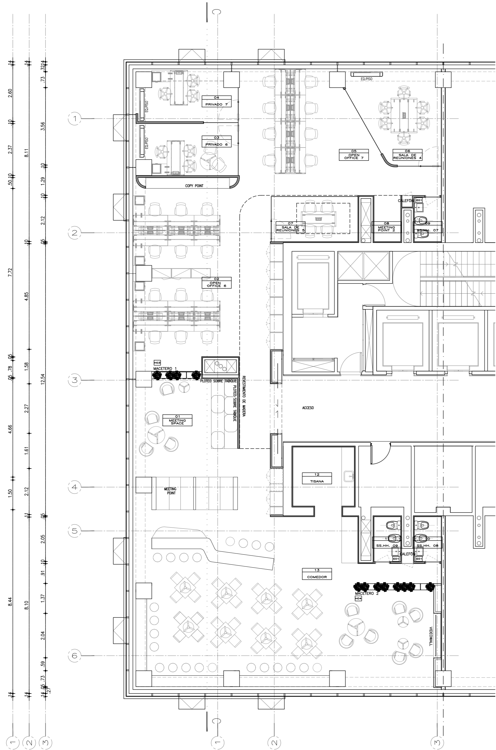
PLANTA ESC 1_100
