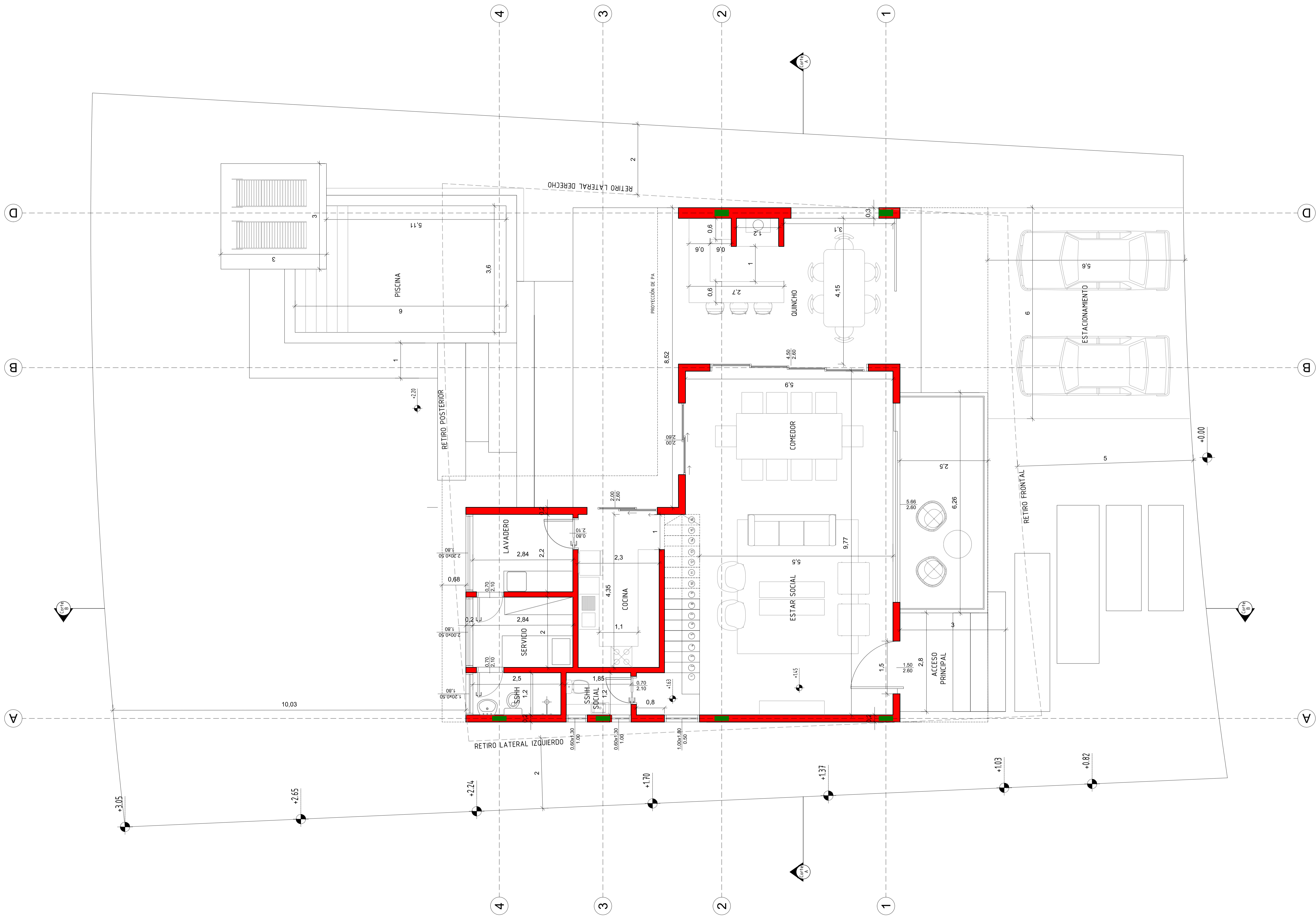
PLANTA BAJA ARQUITECTÓNICA ESC. 1/50
