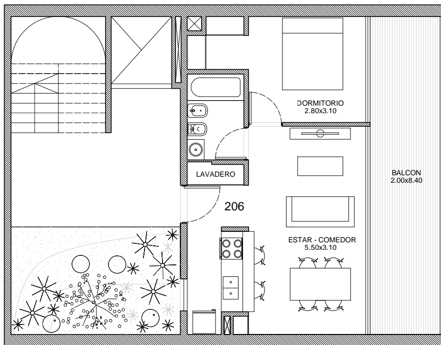
206: 2 AMBIENTES Cubiertos: 43.72m 2 + Balcón: 16.08m 2
